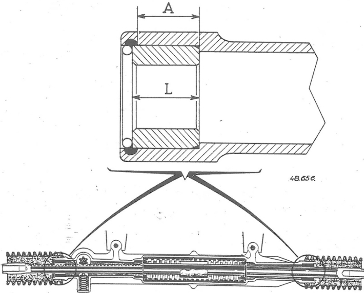
Exemple de bague-palier trop longue, ne permettant pas le montage correct du jonc d'arrêt.
